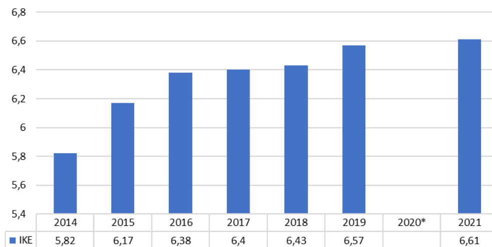
Gambar 2. 6. Grafik Perkembangan Indeks Ketahanan Energi (IKE) Nasional Tahun 2014-2021
