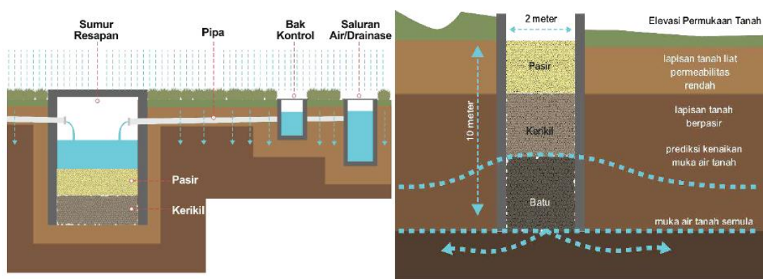
Gambar 30. Ilustrasi Pengembangan Ruang Terbuka Biru – Sumur Resapan
