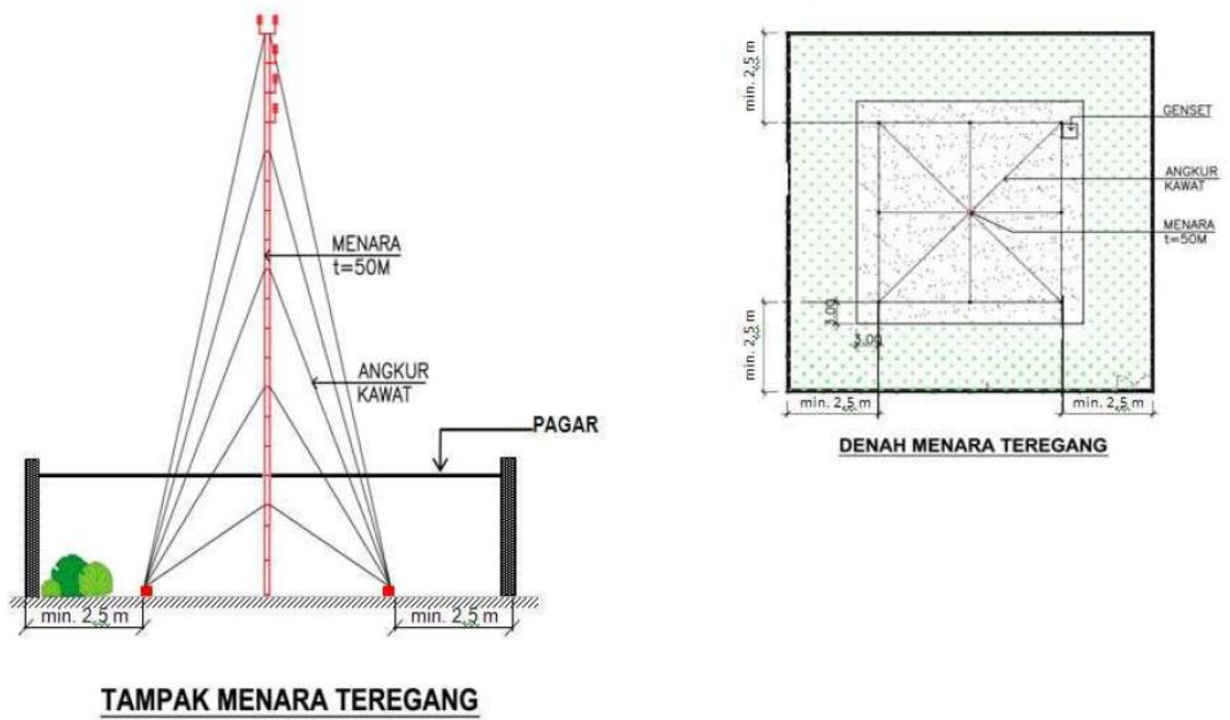
Gambar 7. Ilustrasi Jarak Bebas Menara Tegang Terhadap Bangunan Terdekat
