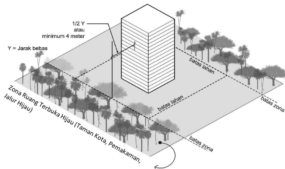
Gambar 36. Ilustrasi Penentuan Jarak Bebas Bangunan Pada lahan perencanaan yang berhimpitan dengan Zona RTH
