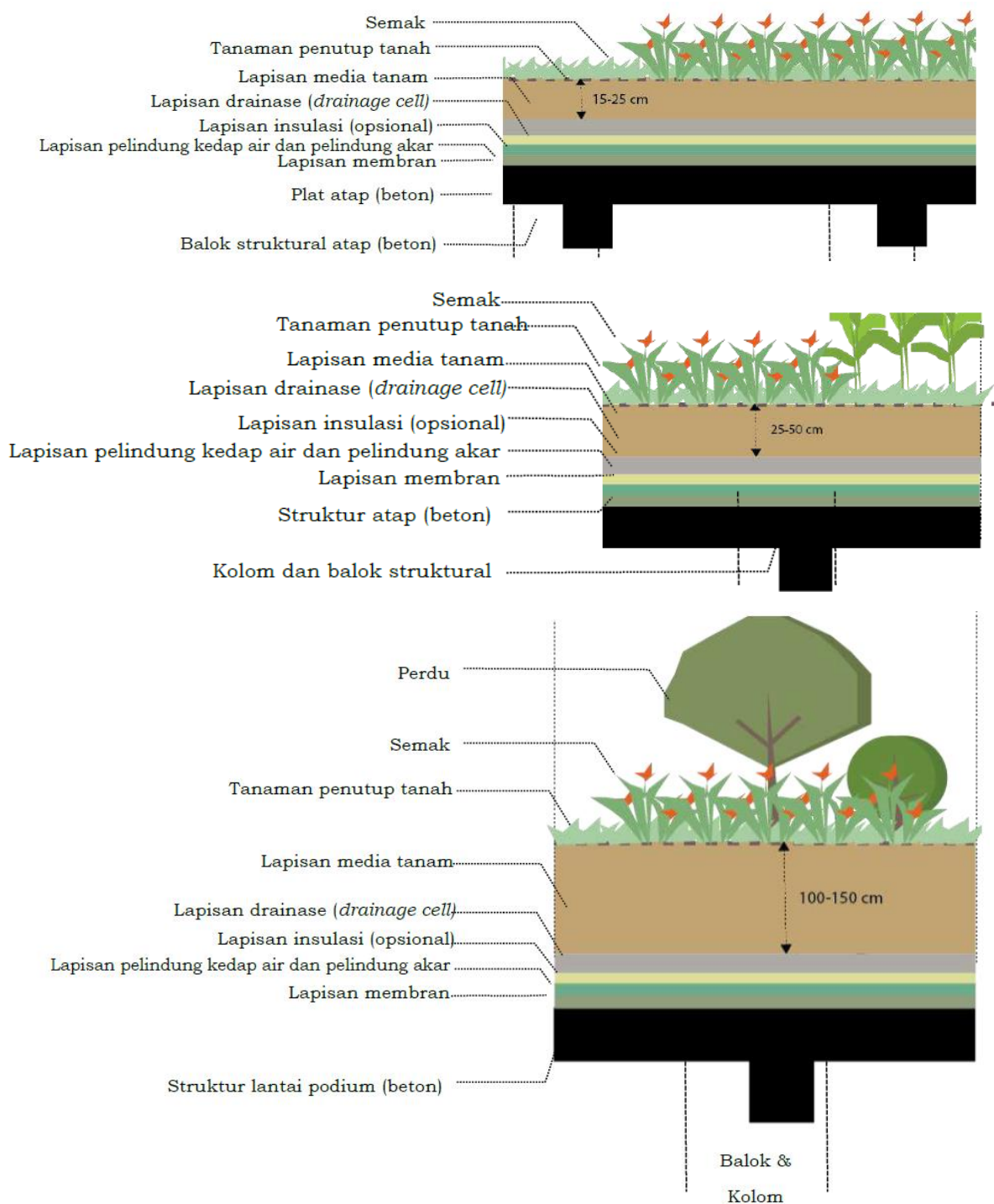
Gambar 17. Ilustrasi Taman Podium Intensif
