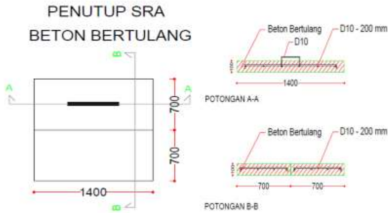
Gambar 4.64. Desain tutup SRA tipe tertutup
