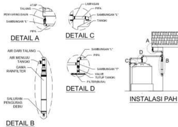
Gambar 4.71. Detail Komponen Rainfilter pada IPAH
