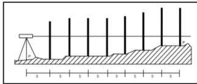
Gambar 6. Profil memanjang
