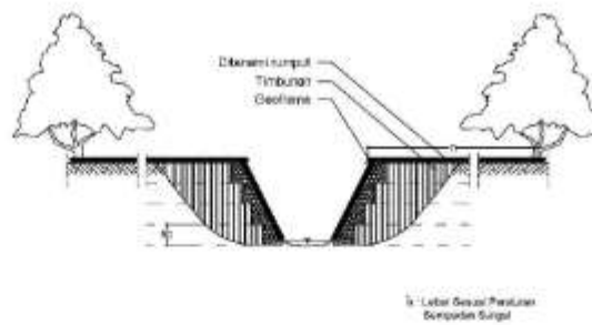
POTONGAN A-A SKALA 1:70
