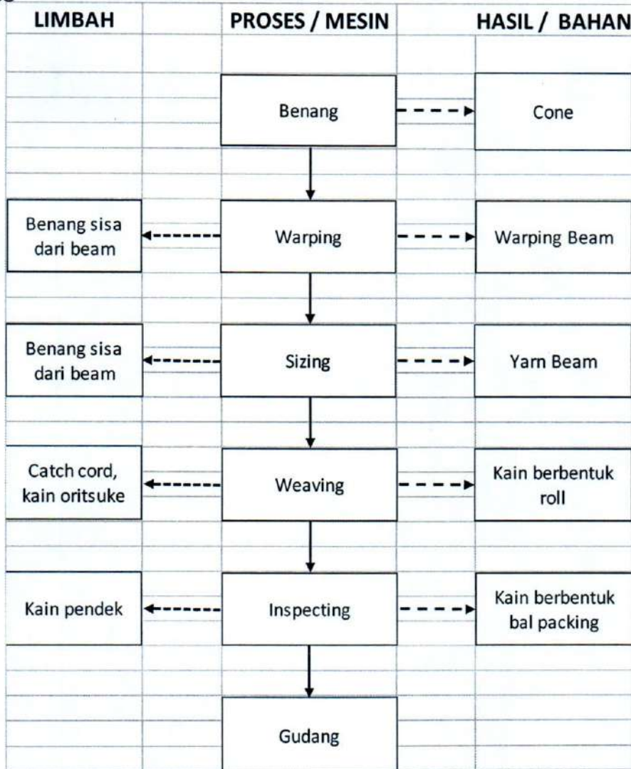
Gambar 2 – Bagan Alir Proses Produksi Industri Pertenunan yang Menggunakan Alat Tenun Mesin
