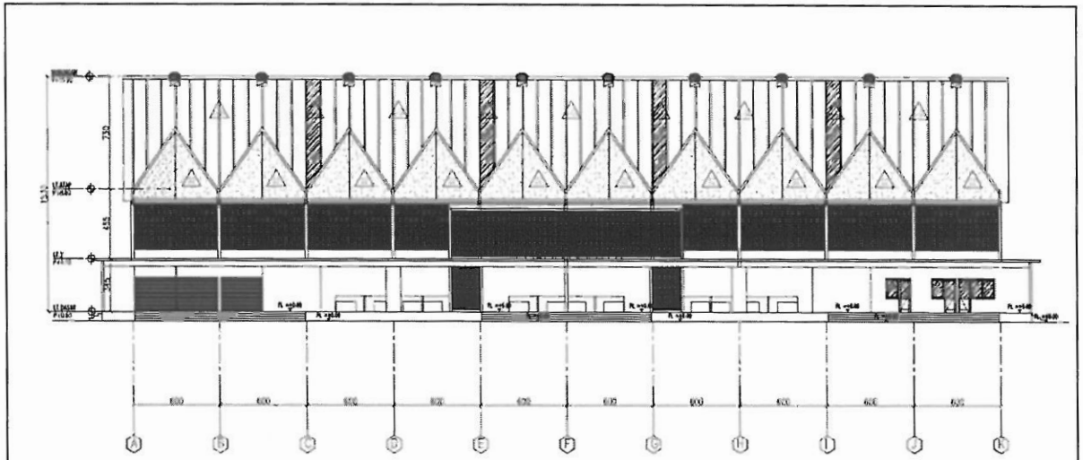
TAMPAK DEPAN/SELATAN/UTARA (VIEW A) SKALA 1 : 200
