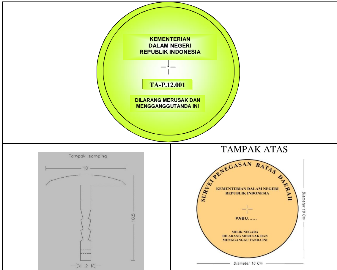
Gambar 12 Konstruksi Brass Tablet
