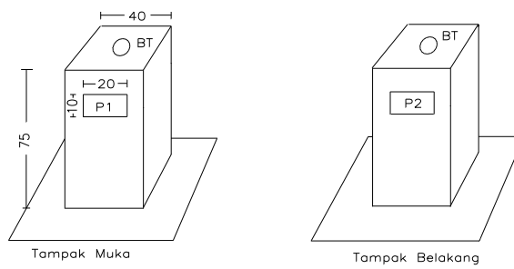
Gambar 9 Konstruksi Pilar Tipe A
