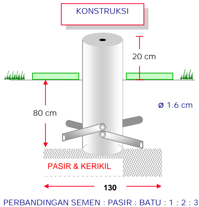
Gambar 17 Bentuk dan Dimensi Pilar Titik Bantu
