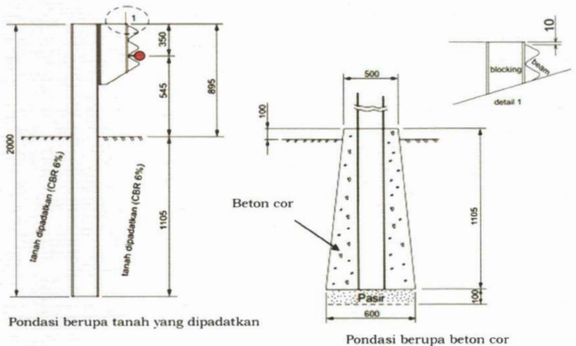
Detail Pondasi Pagar Pengaman Semi Kaku Jenis Lempeng Balok Tiga Lengkung ( Thrie Beam )
