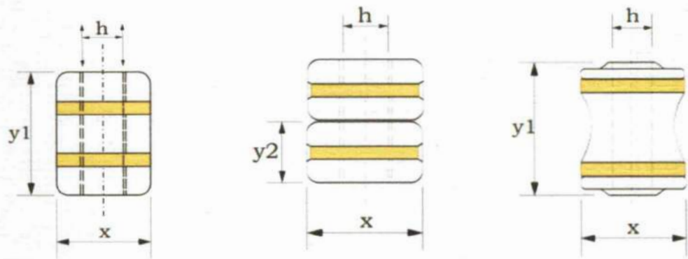
Gambar 36 Jenis-Jenis Bentuk Penampang Roller
