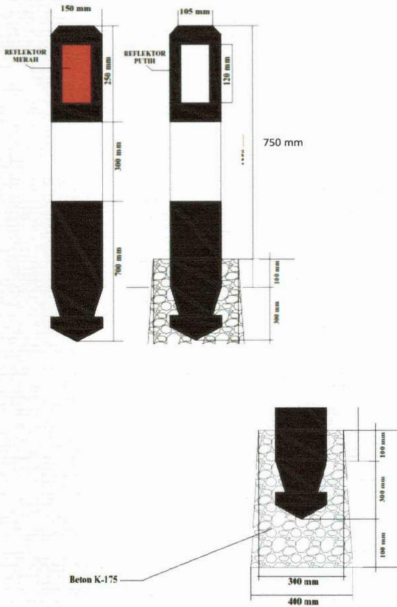
Gambar 53 Spesifikasi Delineator Plastik
