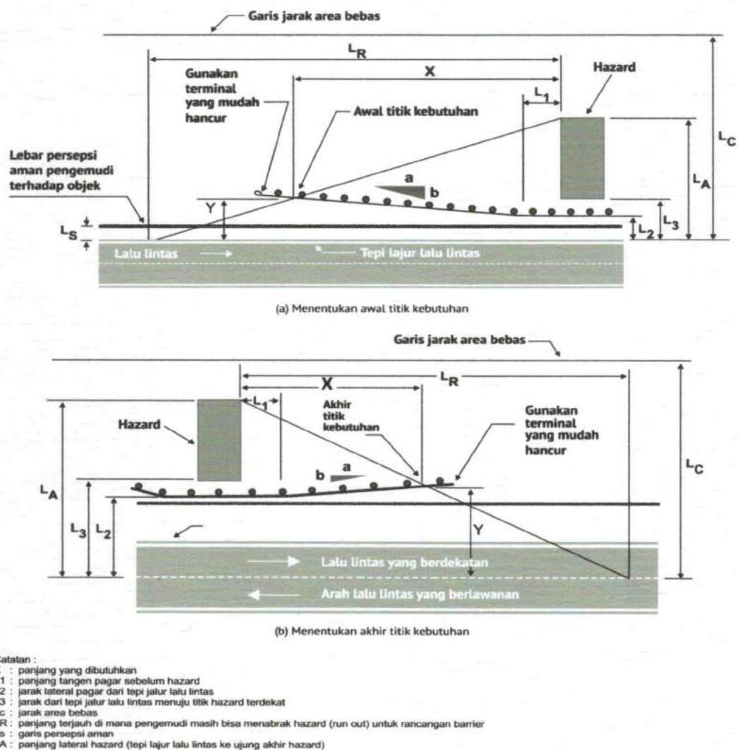
Gambar 17 Panjang Kebutuhan Pagar Pengaman pada Sisi Jalan Lurus
