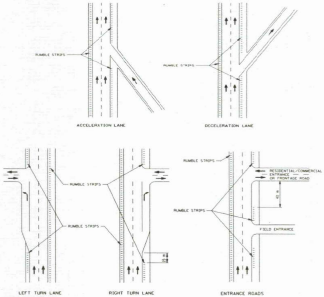
Gambar 63 Penempatan Shoulder Rumble
