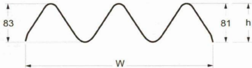
Gambar 22 Penampang Melintang Lempeng Balok Tiga Lengkung ( Thrie Beam )
