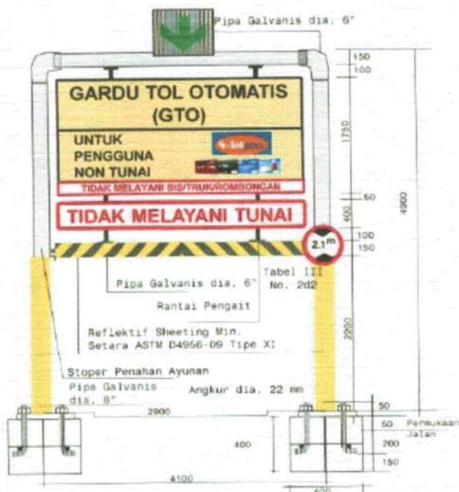
Gambar 4 Alat Pembatas Tinggi dan Lebar
