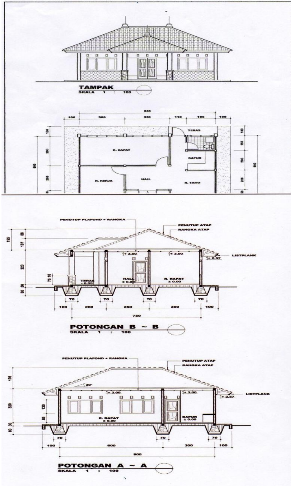
Gambar 38. Contoh Ukuran Bangunan Pos Penyuluhan
