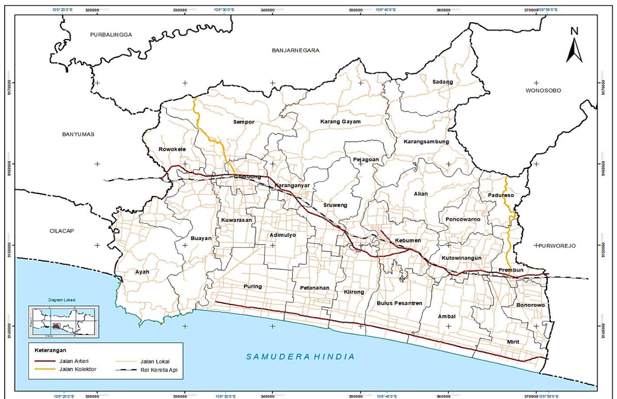
Gambar 2.33 Peta Jaringan Jalan di Kabupaten Kebumen
